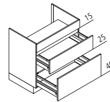
KAK Kochstellenschrank für Muldenlüfter ↳ 60/80/90/100/120 ↓ 80 ↙ 60
