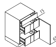
UI Unterschrank
