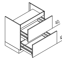
KUZ Kochstellenschrank für Muldenlüfter ↳ 60/80/90/100/120 ↓ 80 ↙ 60
