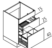
SAKT Spülenunterschrank mit Abfalltrennsystem
