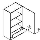
H ASK Aufsatzschrank ↔ 45/50/60 ↓ 115/ ↘ 35
