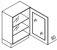
UDDV Unterschrank mit Glasür (programmabhängig) ↳ 40/45/50/60 ↓ 80 ↘ 60/39
