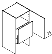
H AL Aufsatzschrank mit Lifttür ↔ 60 ↓ 115/130/145 ↘ 60
