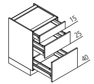
KUAK Kochstellenschrank ↳ 60/80/90/100/120 ↓ 80 ↙ 60
